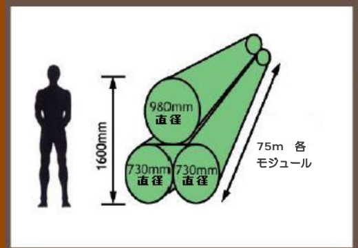
SD 300 3コイル標準システム
