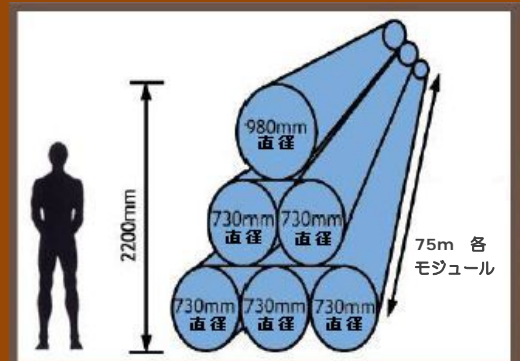
SD 600 6コイル標準システム
